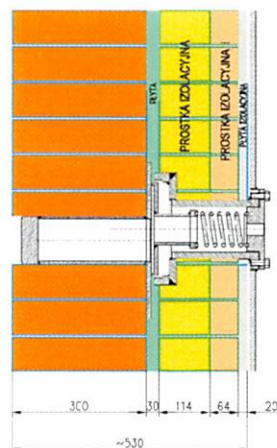
WARIANT 2 PRZY GRUBOŚCI WYMUROWKI 530
