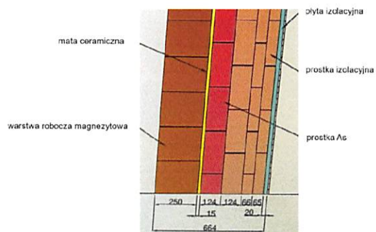
WARIANT 3 GRUBOŚCI WYMUROWKI 664
