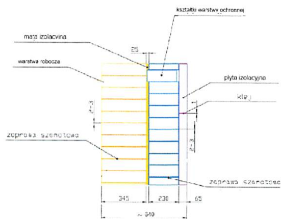
WARIANT 1 PRZY GRUBOŚCI WYMUROWKI 640
